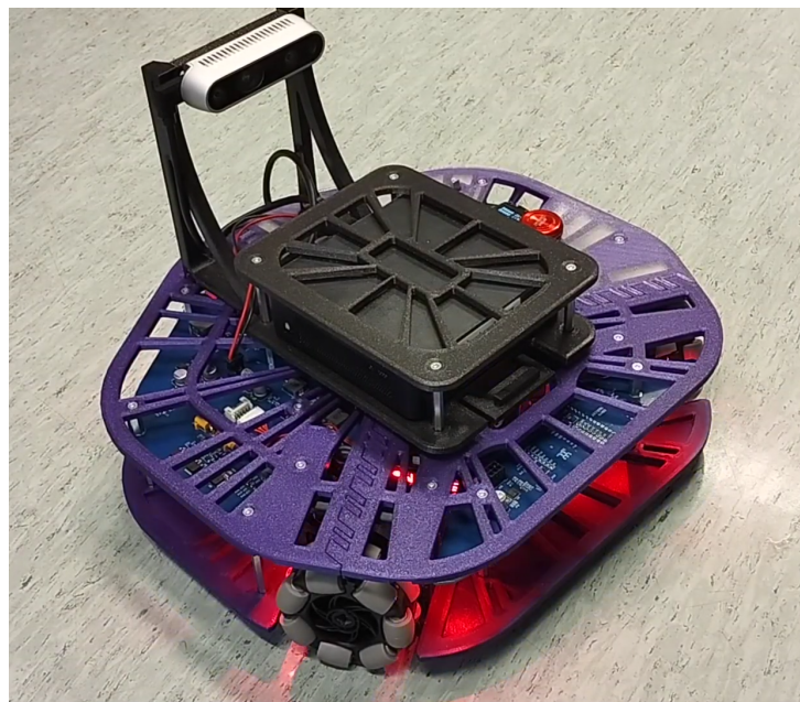
Joonis 5.3: Robotont MOTOR_SPEEDS režiimis vasakule pööramas
