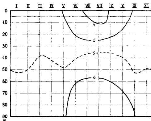
Abb. 13. Isoplethen der Dichte in Utö.
