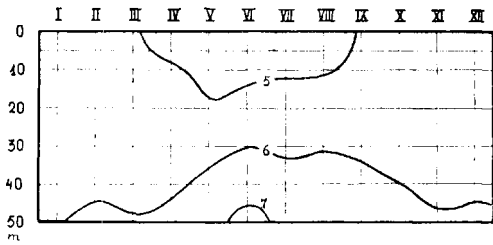
Abb. 9. Isoplethen des Salzgehaltes in Söderskär.
