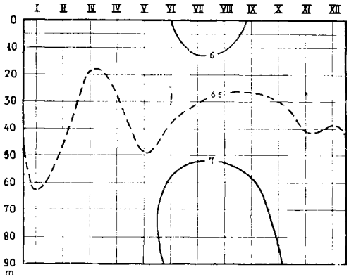
Abb. 7. Isoplethen des Salzgehaltes in Utö.
