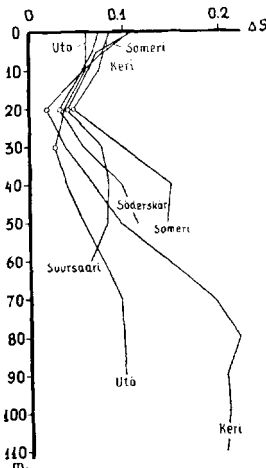
Abb. 11. Die mittlere jährliche Streuung des Salzgehaltes.
