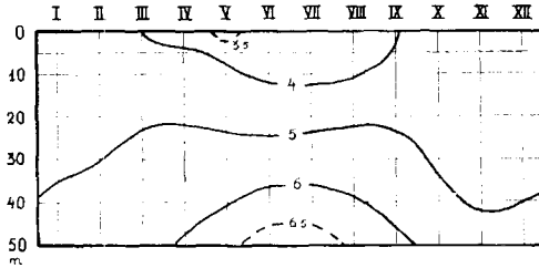
Abb. 10. Isoplethen des Salzgehaltes in Someri.
