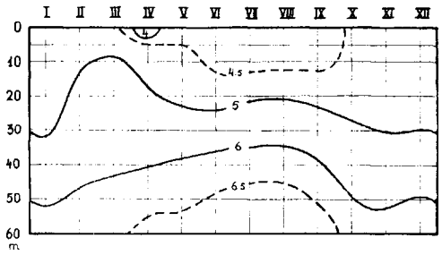
Abb. 8. Isoplethen des Salzgehaltes in Suursaari.
