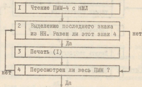
Блок-схема подпрограммы
