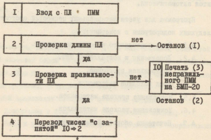
Блок-схема подпрограммы
