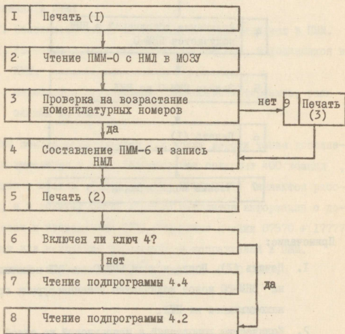
Блок-схема подпрограммы
