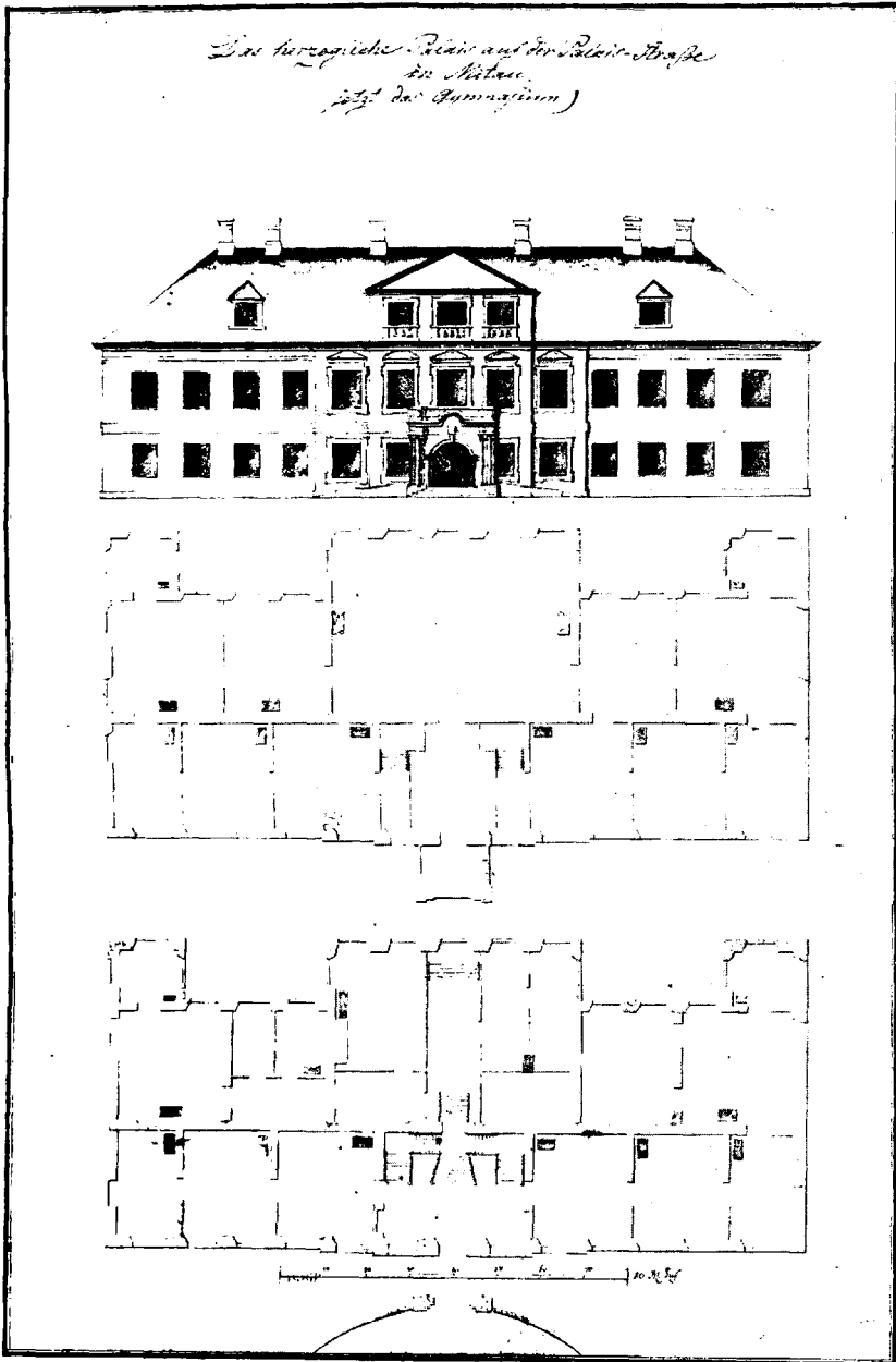
Aufriß und Grundrisse des ehemaligen herzoglichen Palais in Mitau (vgl. dazu S. 103).
