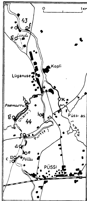
Fig. 3. Aufschlüsse der Tallinna-Serie am Purtse-Fluss in der Umgebung von Lügänuše und Püssi: 43 e, f — Aufschlüsse der Aseri-Stufe. 43 g, 44 h — Aufschlüsse der Lasnamäe-Stufe. 44 c, d, e, f, g, h — Aufschlüsse der Uhaku-Stufe und der hangenden Schichten.
