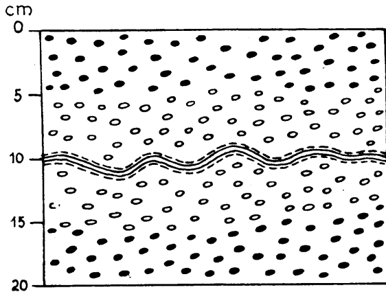
Fig. 1. Abgerutschter Block der Aseri-Stufe aus Lahepere (?): grauer, harter Kalkstein mit vielen Eisenooiden. Den Block durchzieht eine schmale, mit kristallinischem Kalzit gefüllte Spalte, an deren Rändern reichlich Pyrit auskristallisiert ist. Das Pyrit hat sich hier während des Reduktionsprozesses angehäuft, während die Eisenoide in der Nähe des Spalts ihren Eisengehalt verloren und sich auf diese Weise in weisse Ooide verwandelt haben.
