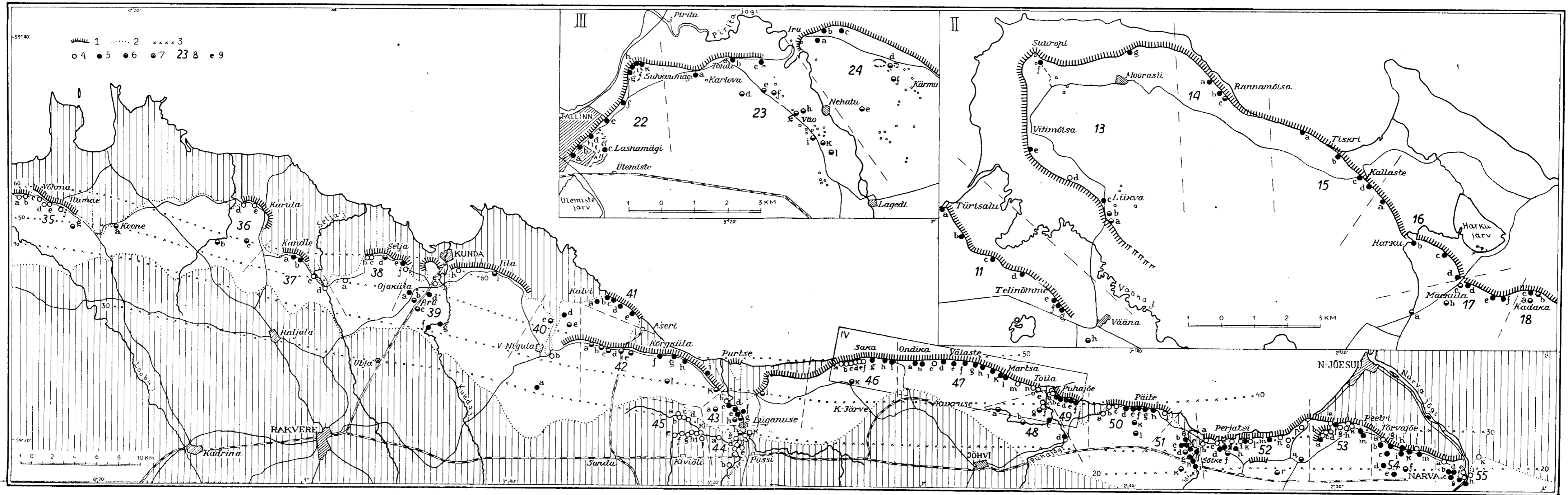
Die Aufschlüsse und das Anstehende der Tallinna-Serie (s. Text S. 10—34 u. S. 35—38). Massstab 1:252.000.
