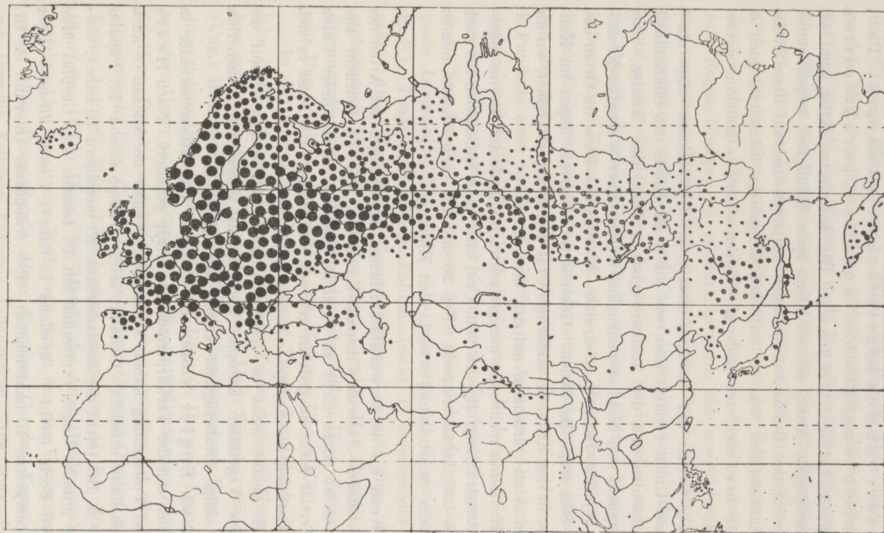
Fig. 27. Die Verbreitung der konstanten Arten der Galeobdolon-Asperula-Asarum -Union.
