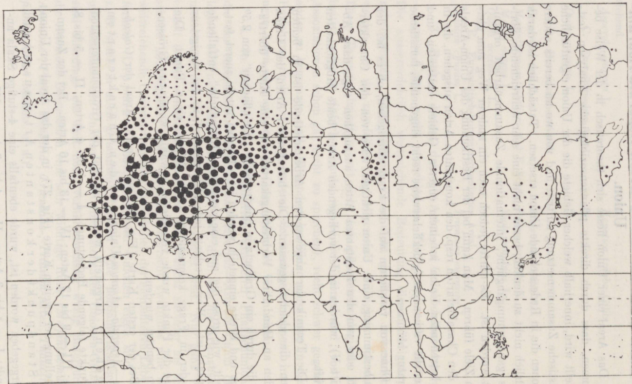
Fig. 26. Das Areal der Galeobdolon — Asperula — Asarum -Union. • 1 bis 4, • 5 bis 8, • 9 bis 12, ● 13 bis 16 Charakterarten.
