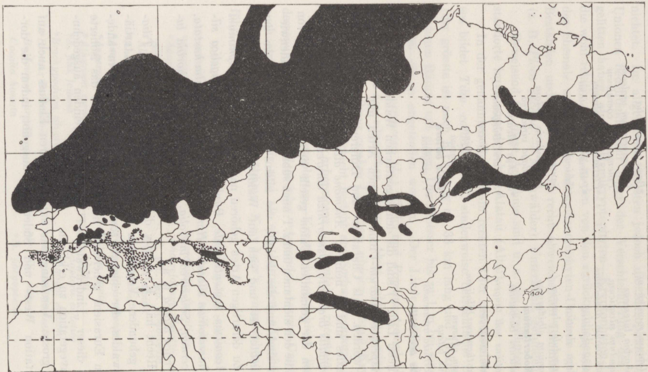
Fig. 28. Maximale Ausbreitung der diluvialen Eisdecke (schwarz) nach De Geer, Grahmann, Sobolew, Bubnoff, Obrutschew, Tolmatschew u. a. und die mutmasslichen Erhaltungsgebiete der Buche im Diluvium nach Lämmermayr (punktiert).
