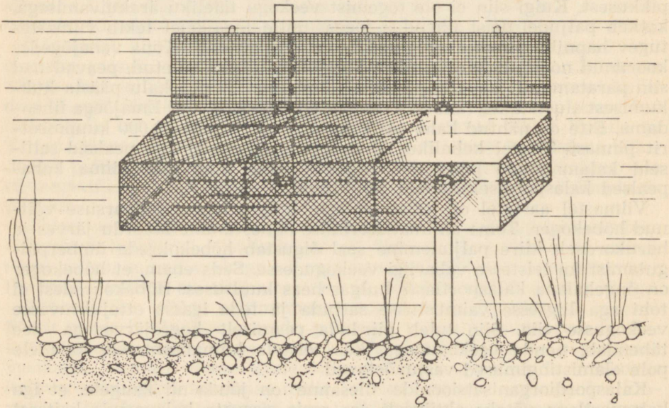
«Rummu inkubaator» — kastikujuline haudeparaat kalamarja inkubeerimiseks looduslikes tingimustes. (Pildil on inkubaator näidatud maimude vetelaskmise asendis — avatud kaanega.)
