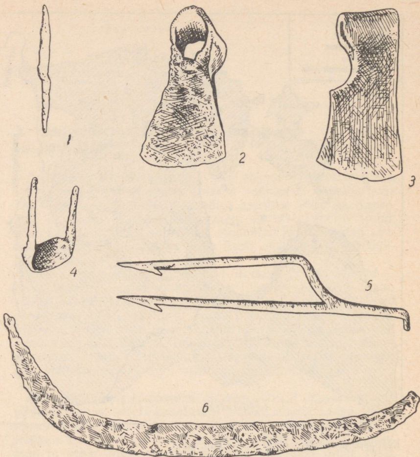
Rauast tööriistu XI—XII sajandist. 1 — nuga; 2 ja 3 — kirved; 4 — voolmed; 5 — poolik ahing; 6 vikat.
