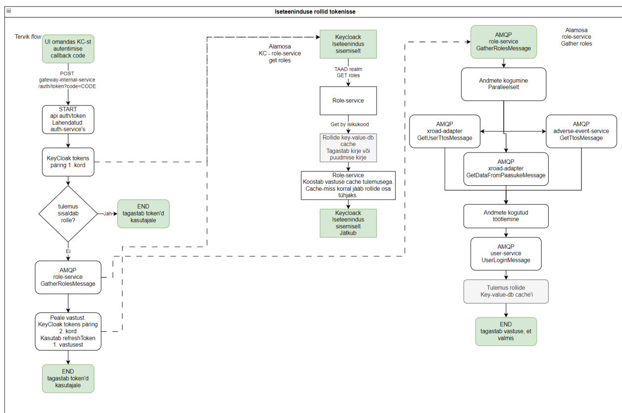
Joonis 6. Iseteeninduse sisselogimise voog
