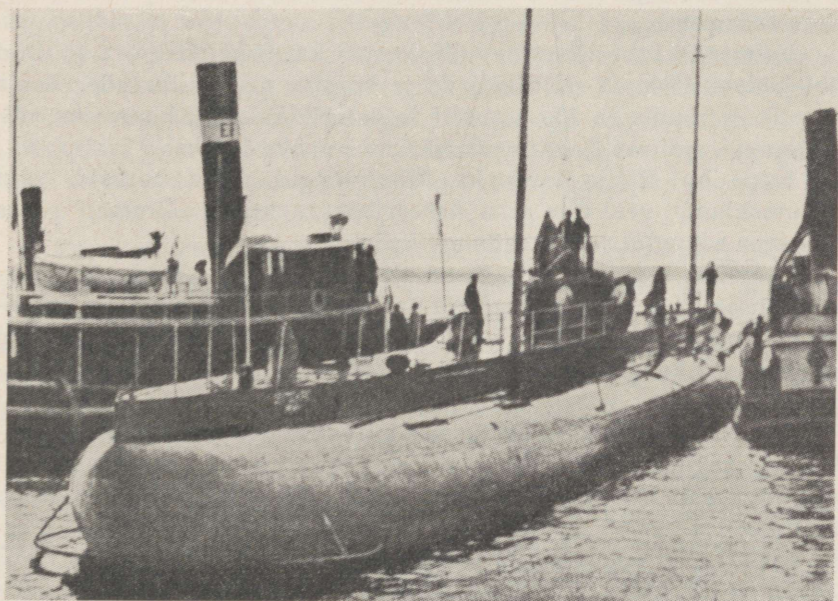
Saksa kauba-allveelaev „Deutschland“ Baltimore sadamas.
